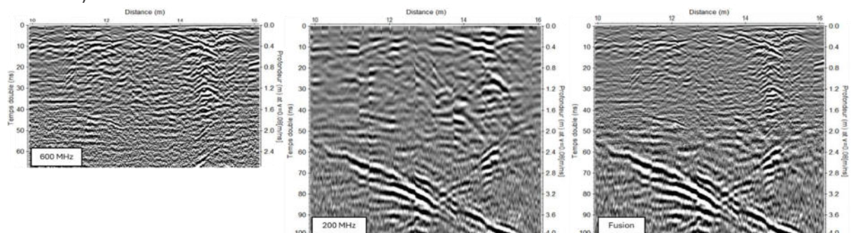
Fig. 2 - Extrait de radargrammes en piédroit-voûte (1h), traités avec la partie de l'antenne de fréquence centrale 600 MHz (à gauche), et de 200 MHz (au centre) puis après fusion de ces deux types de données (à droite).
