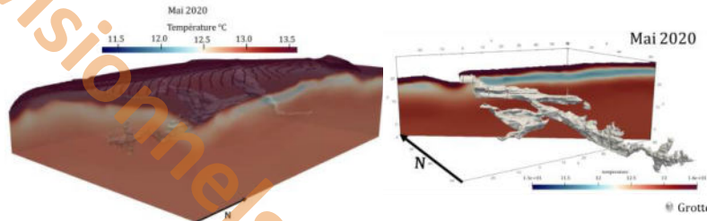
Fig. 3 – (1) Champ de température simulé dans le massif et (2) coupe transversale du champ de température pendant le mois de mai 2020. La cavité est représentée en gris.
