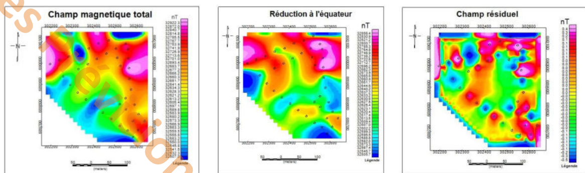
Figure 2 : Cartes magnétiques de la décharge d'Agoé-Nyivè
