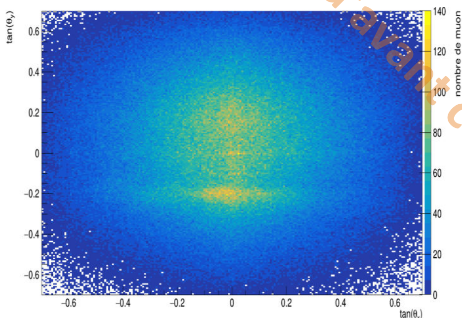
Fig. 3 -Carte du nombre de muons obtenu lors de la campagne de May-sur-Orne
