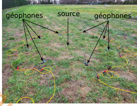
FIGURE 1 – Configuration expérimentale
