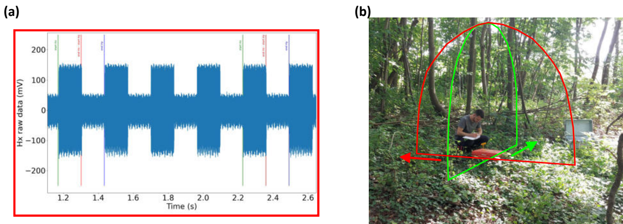
Fig. 1 – Une source composée de deux dipôles magnétiques : (a) extrait d'une séquence de mesures ; (b) photo de l'émetteur EH4 sur le terrain.
