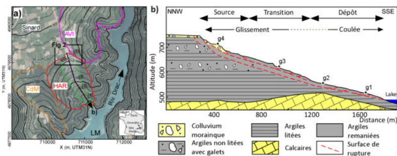
Fig. 1 – Présentation du site d'étude. a) Localisation. AVI : glissement d'Avignonet ; HAR : glissement d'Harmalière ; CdM : glissement du Champ du mouton. LM : Lac de Monteynjard. g0-g4 : stations GNSS. b) Coupe géologique synthétique au centre du glissement (localisation sur la Figure 1a) et mécanismes de déformation associés.
