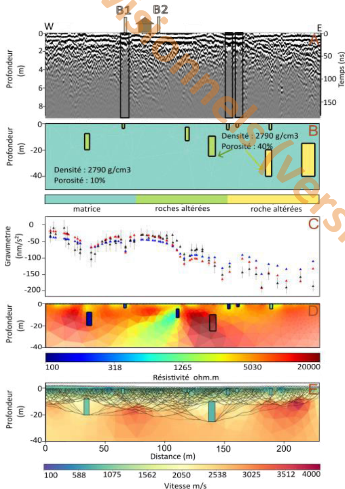
Fig. 2 – Résultats des inversions des données de terrain pour les quatre profils étudié. (A) Données de terrain géoradar, les encadrés noirs sous les trois zones de plus fortes atténuations. (B) Modèle initial utilisé pour réaliser le modèle synthétique, les valeurs de porosité et densité sont acquises sur des échantillons de roches. Le bleu représente la matrice, les roches altérées sont en vert et jaune, les structures vertes sont utilisées pour réaliser le mesh pour les inversions contraintes ERT et SRT, les structures jaunes sont ajoutées pour générer les données synthétiques gravimétriques. (C) Données gravimétriques de terrain en noir, les données synthétiques sont en bleu et rouge. En bleu les milieux sont entièrement saturés en eau et en rouge non saturés. (D) Résultats de l'inversion contrainte des données de terrain ERT. (E) Résultats de l'inversion contrainte des données SRT de terrain.
