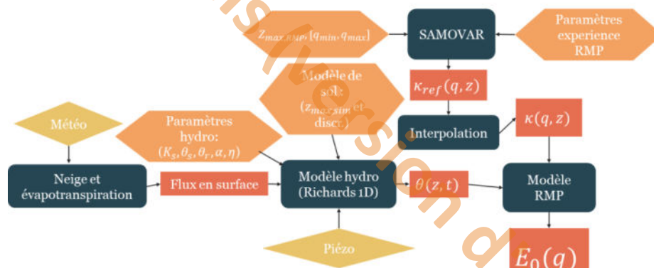
Fig. 2 – Schéma du modèle hydrogéophysique couplé.
