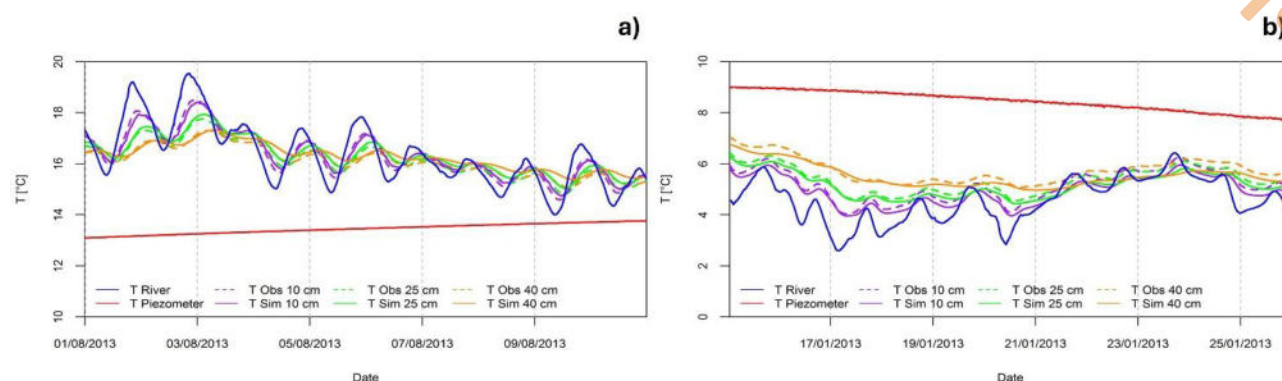
Fig. 3: Comparaison entre les températures simulées (trait continu) et les températures observées (trait pointillé) à différentes profondeurs de la section 2 : a) Calibration dans le cas d'une infiltration et b) Validation dans le cas d'une exfiltration
