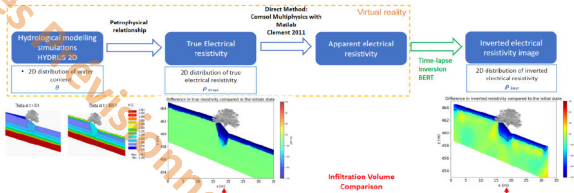
Fig. 1 –Aperçu de la stratégie numérique utilisé pour évaluer les différentes stratégies d'acquisition de TL-ERT.
