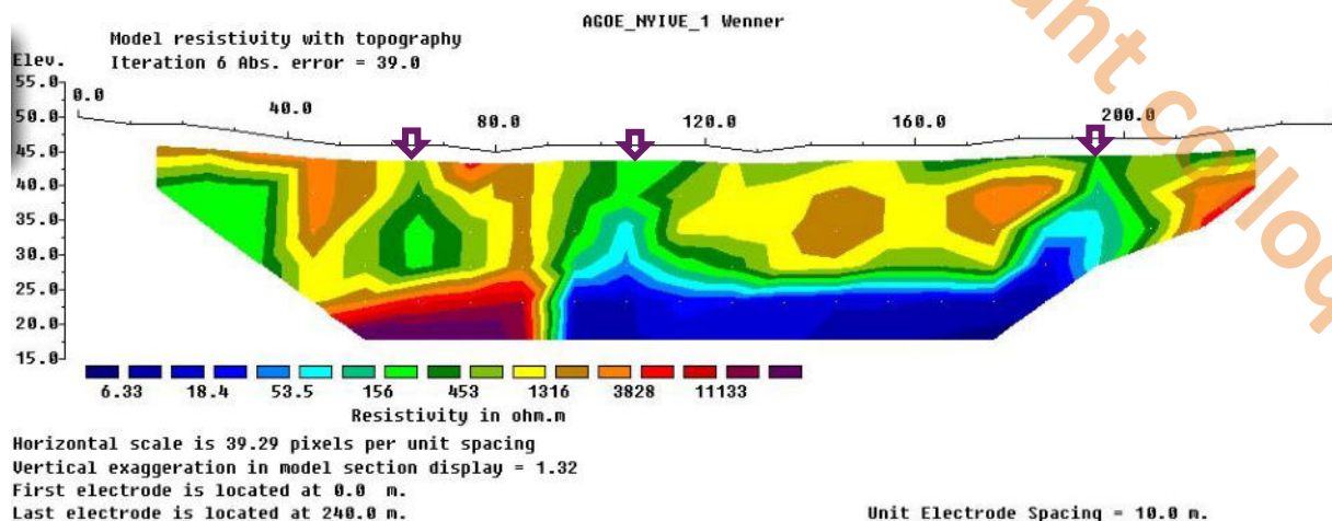
Figure 3 : Section ERT sur la décharge d'Agoe-Nyivè
