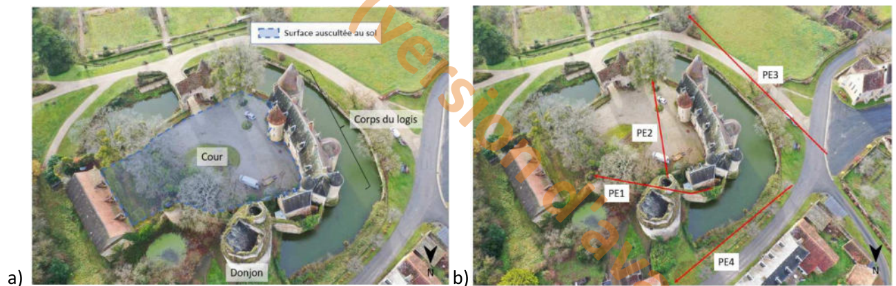
Fig. 1 - Localisation des investigations géophysiques a) Géoradar zone bleue); b) Tomographie électrique (lignes rouges)
